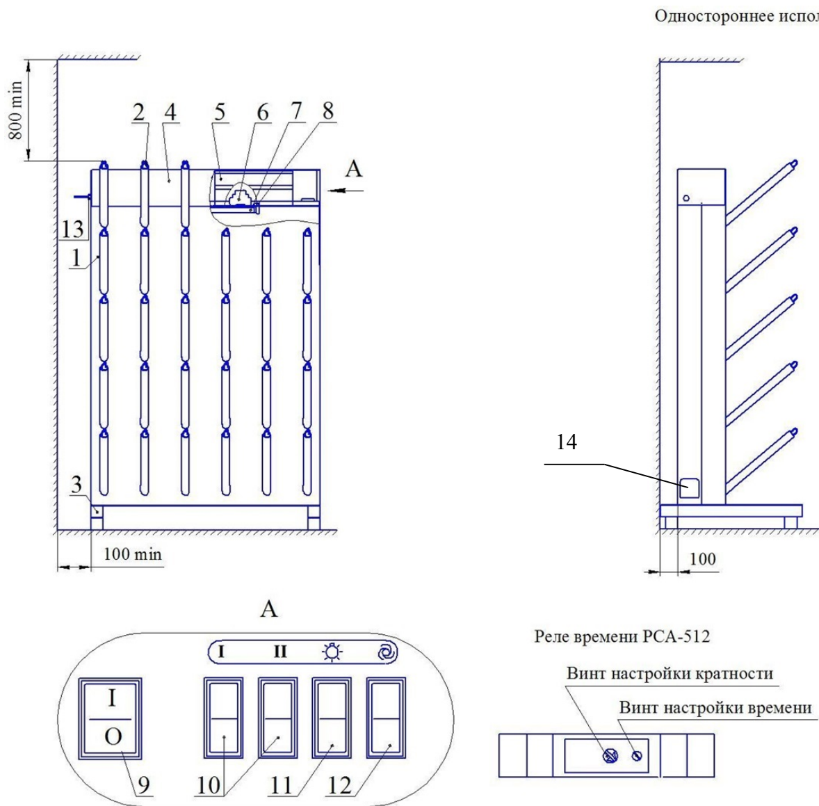
Рисунок 2-Сушилка для обуви СОМ -40-01 односторонняя
