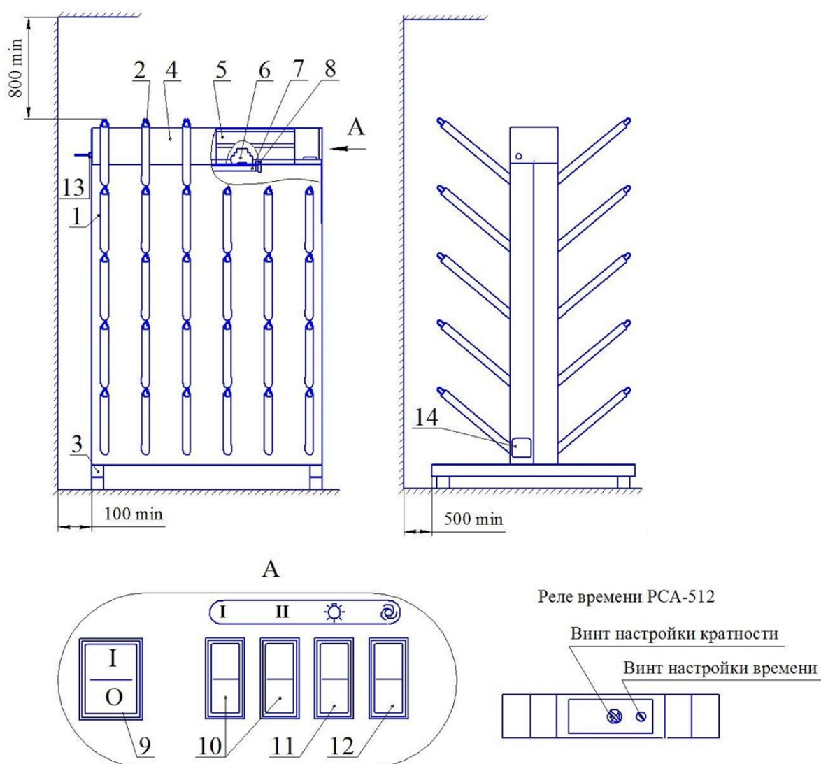
Рисунок 1-Сушилка для обуви СОМ -40 двухсторонняя
