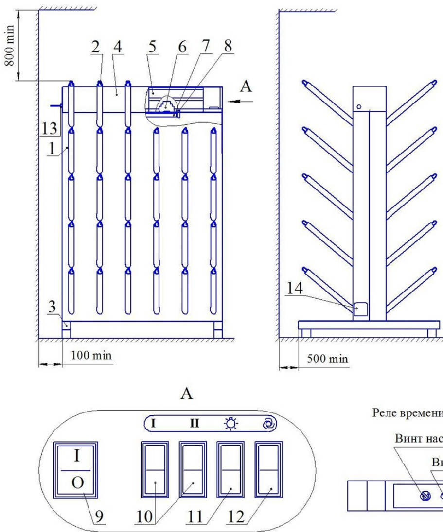
Рисунок 1-Сушилка для обуви СОМ -40 двухсторонняя
