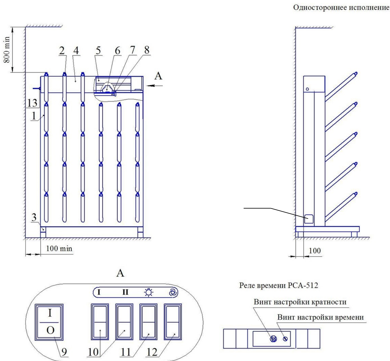
Рисунок 2-Сушилка для обуви СМ -40-01 односторонняя
