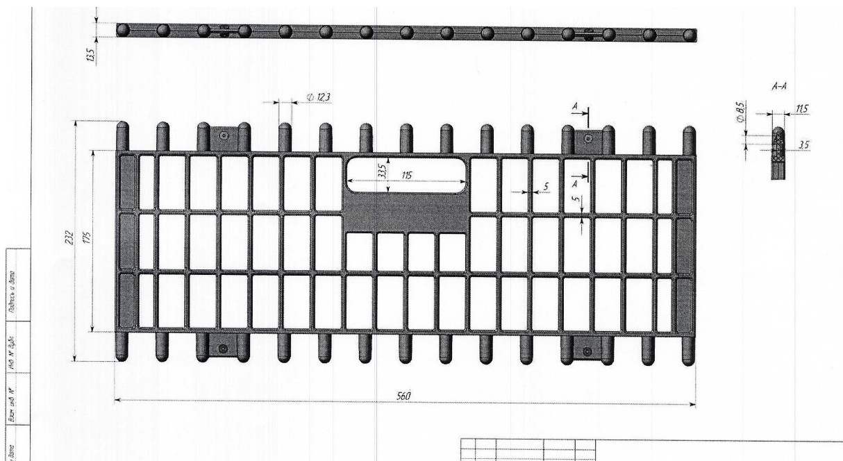
Чертеж короткой стенки ящика, ручки и фиксатора
