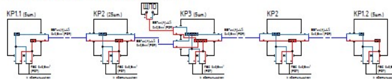
Схема соединений в распределительных коробках КР1-КР3
