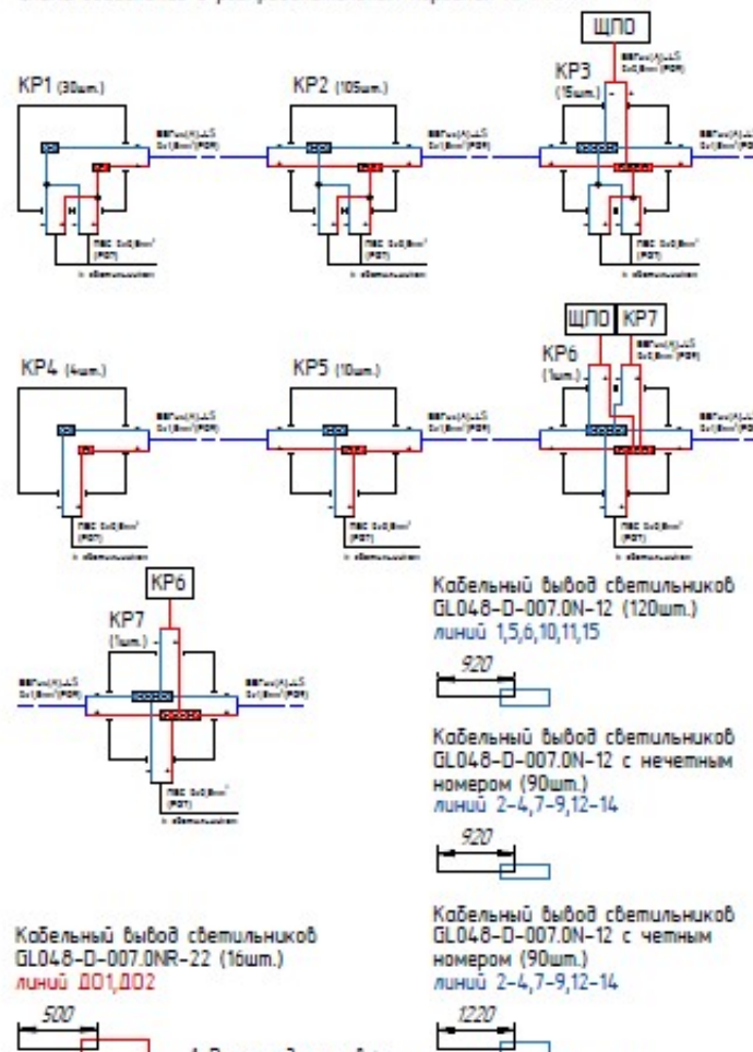
Схема соединений в распределительных коробках КР1-КР7
